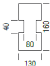
DIMENSIONE PALO
